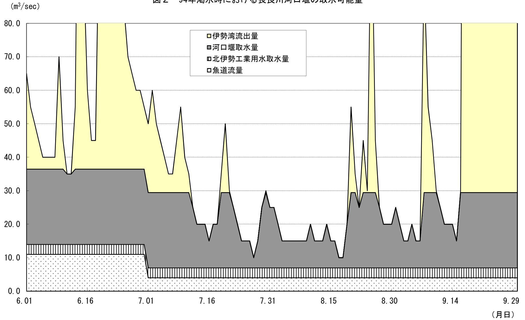
図2 94年渇水時における長良川河口堰の取水可能量
