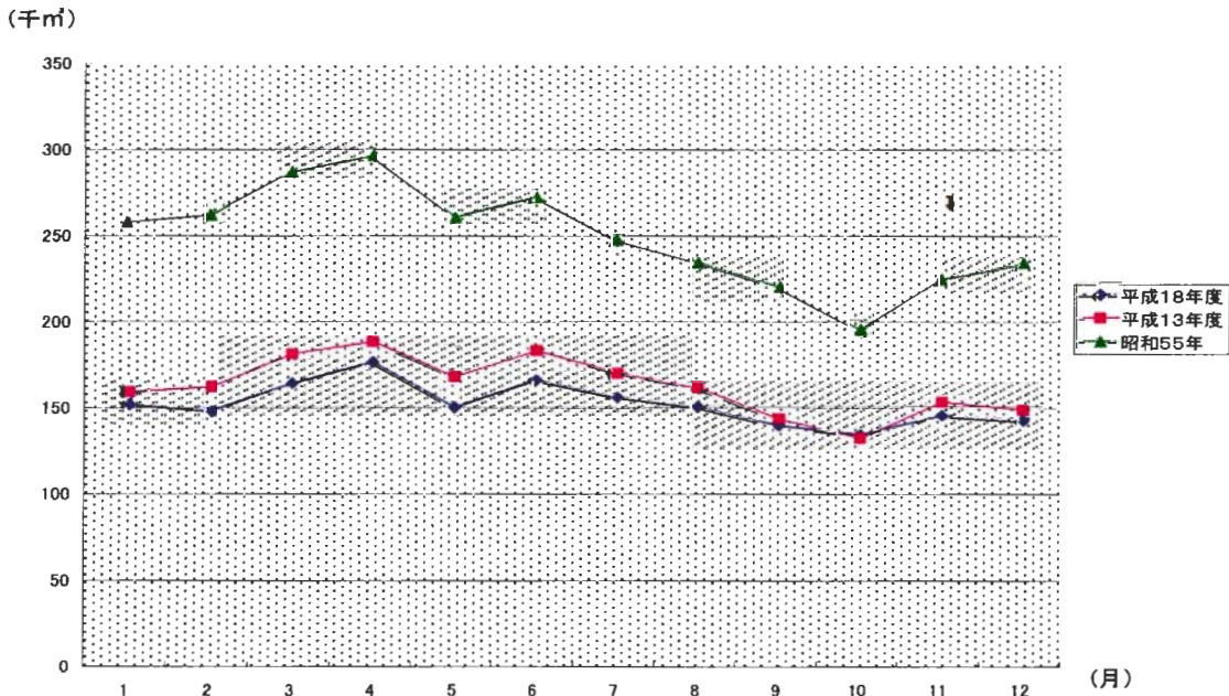
図10-2 大垣市内の年度別・月別地下水揚水量
