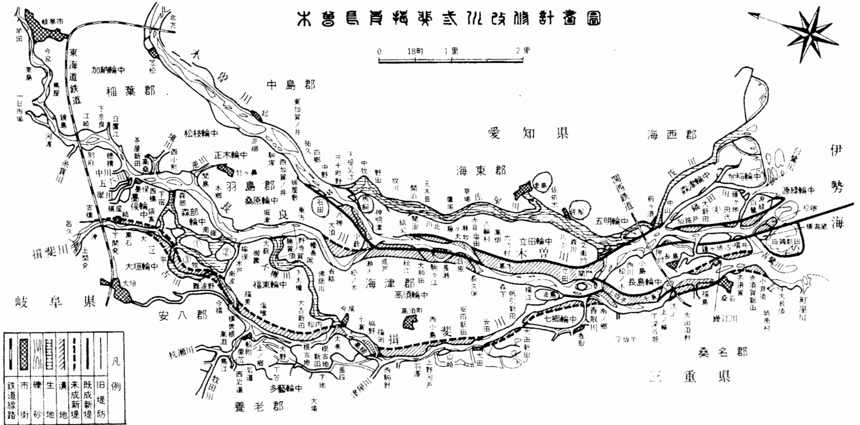
木曾長良揖斐三川改修計画圖
