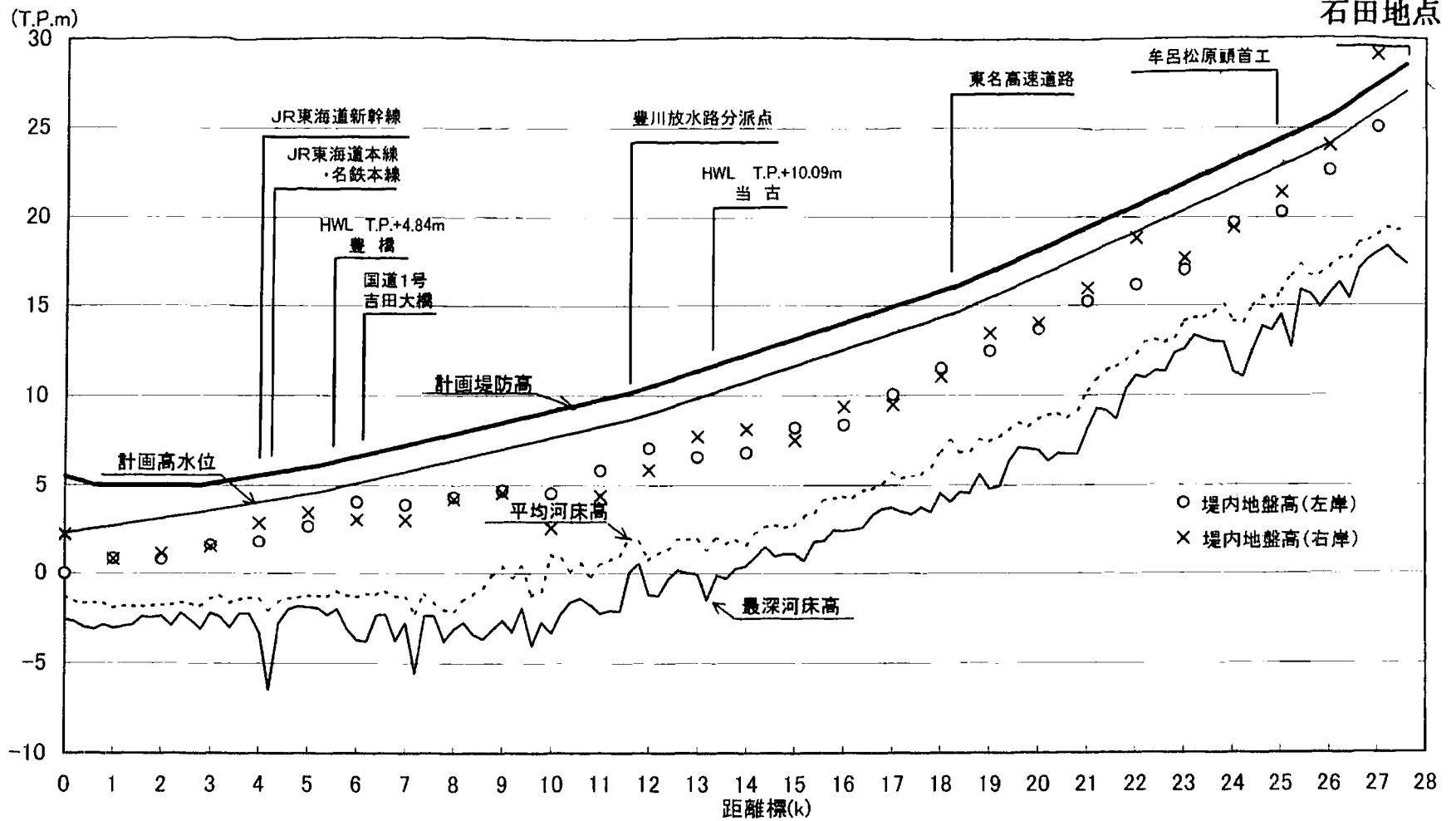
付図2 豊川の河川縦断図
