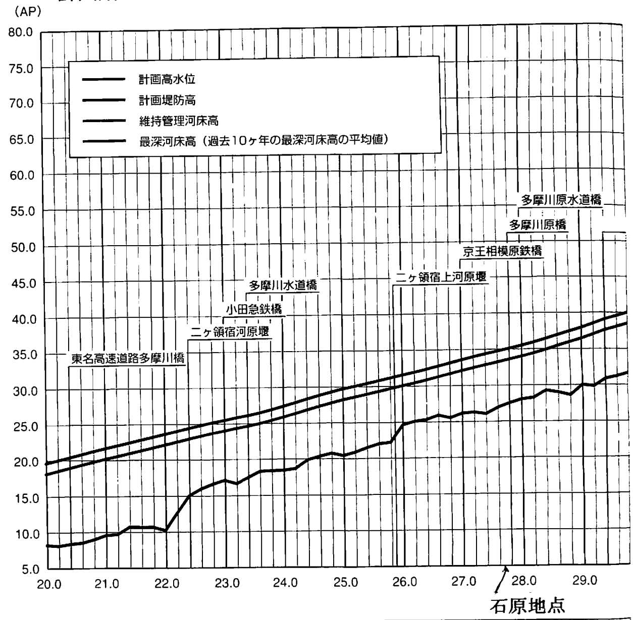
計画諸元表・多摩川 (20.0k ~ 39.8k)
